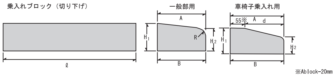
斜ブロック（左右）
